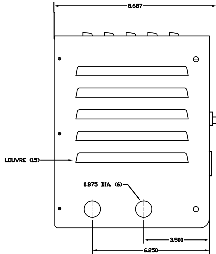
LEFT SIDE
